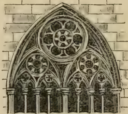
(دائرة بیضیه)
